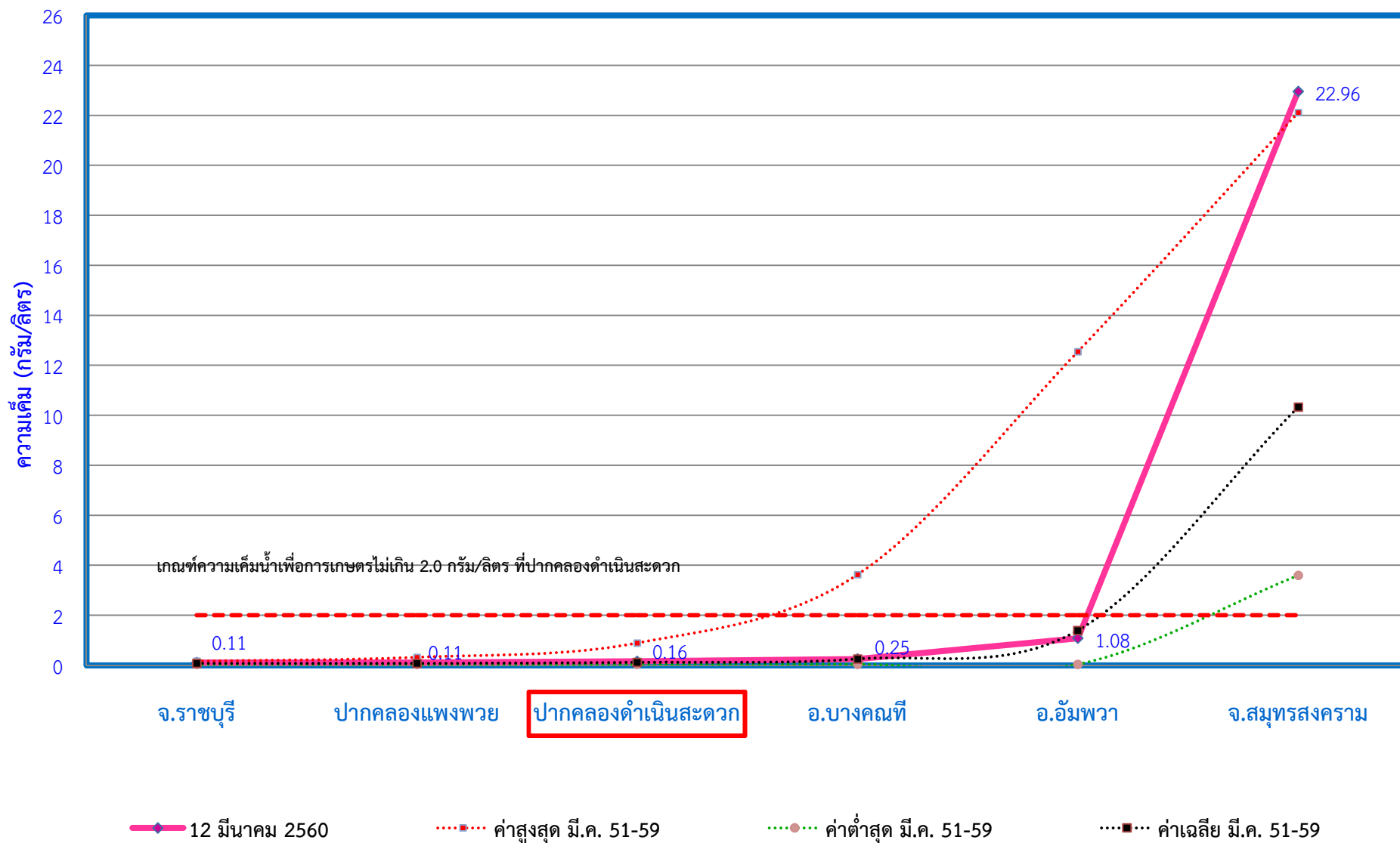
ค่าความเค็มในแม่น้ำแม่กลอง วันที่ 12 มีนาคม 2560
